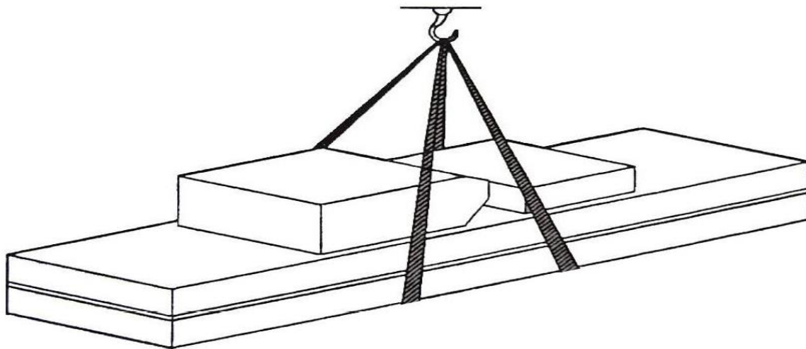
Рис. 1 Стрповка оборудования
